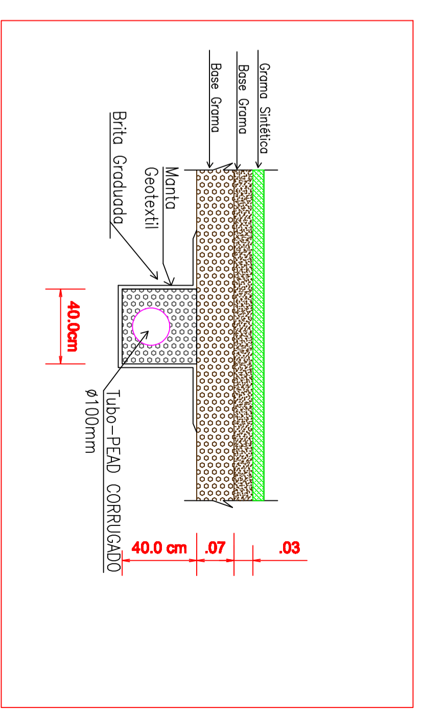
DETALHES - DRENAGEM SEM ESCALA
